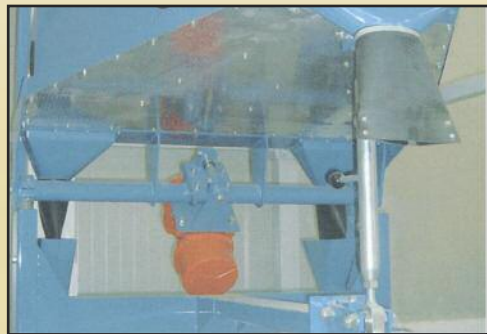
Spietatrice per caffè verde Destoner for raw coffee
